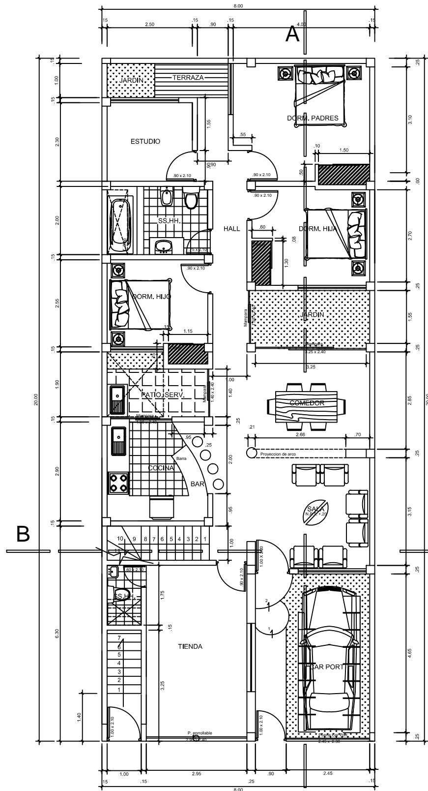
PRIMERA PLANTA
