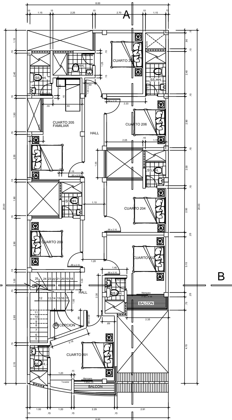
2°-3°-4° PLANTA
