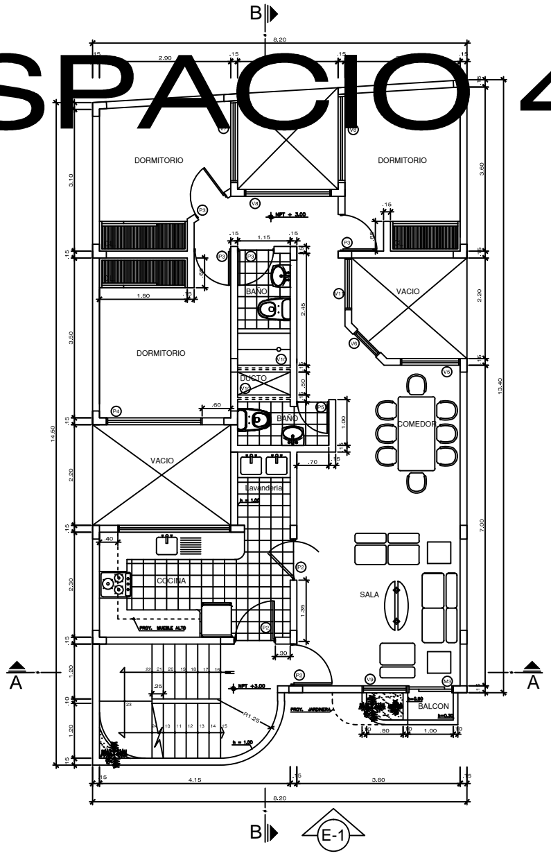
PLANTA TIPICA 2do, 3er, 4to, PISO ESC.: 1/50
