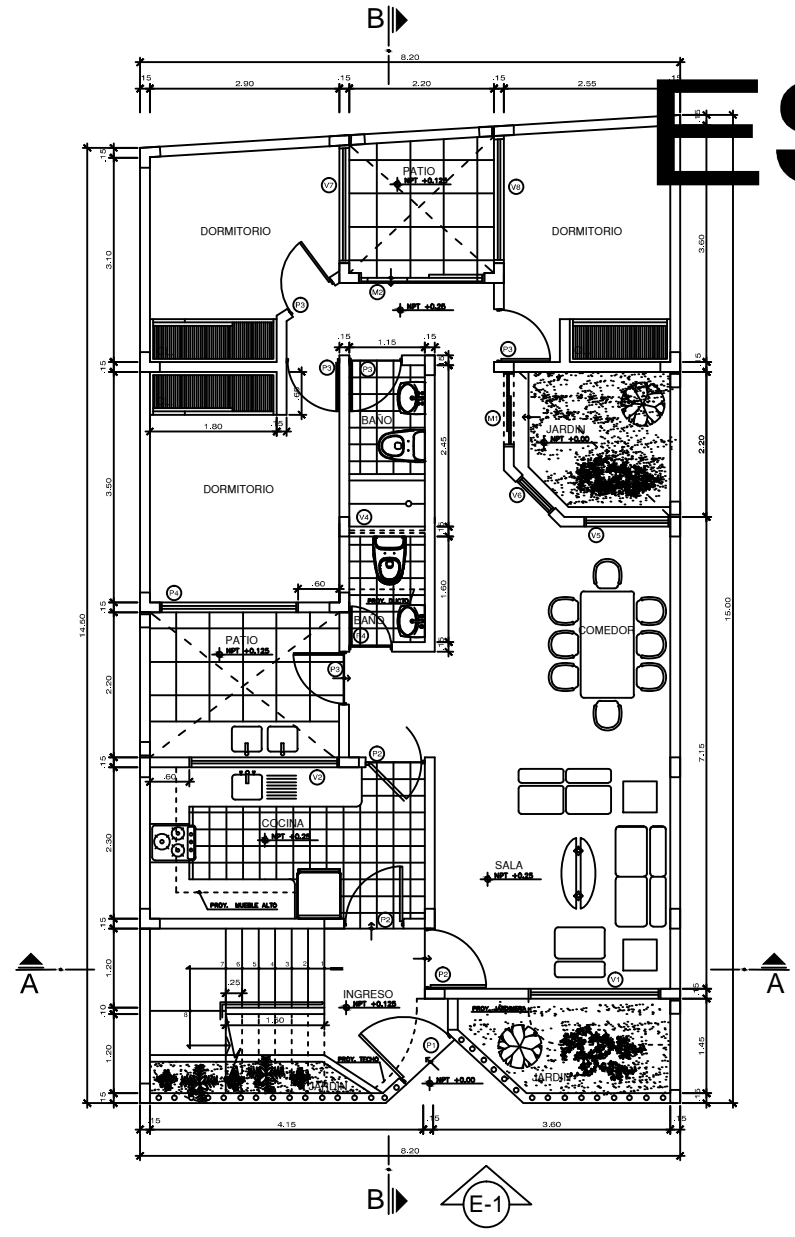
PLANTA 1er PISO ESC.: 1/50
